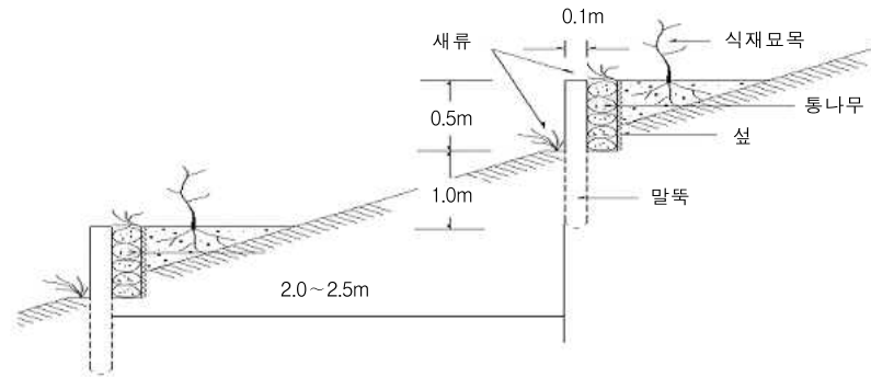
<통나무울짙엮기 예시>
